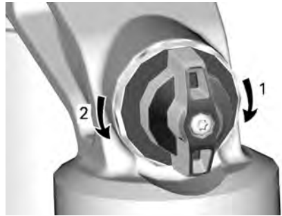
SITUAZIONE TIPICA - REGOLAZIONE CROSSOVER - AMMORTIZZATORE POSTERIORE
