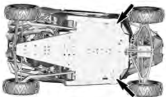
POSIZIONI DEL MARTINETTO - LATO ANTERIORE DEL VEICOLO
