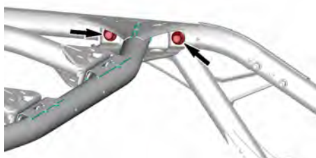
FIXATIONS SUPÉRIEURES ARRIÈRE
