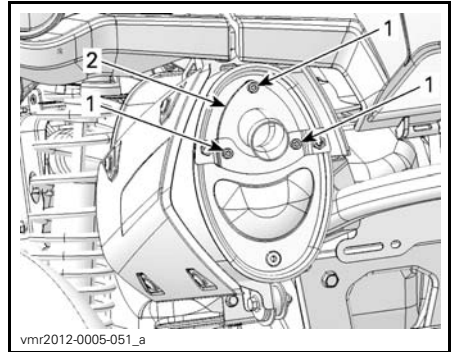
TYPIQUE - RETRAIT DU TUYAU ARRIÈRE
