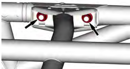
TUERCAS CENTRALES LATERALES — TÍPICAS
