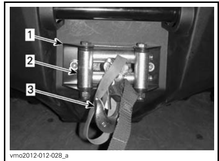
1. Treuil 2. Rouleau pour guide-câble 3. Crochet
