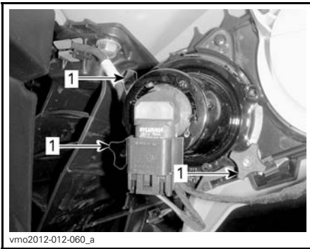
RÉGLAGE DES FEUX DE ROUTE 1. Boutons de réglage
