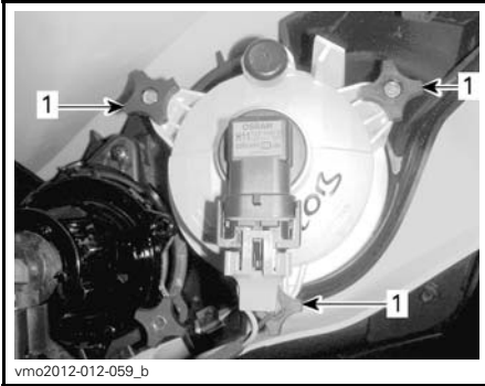
RÉGLAGE DES FEUX DE CROISEMENT 1. Boutons de réglage
