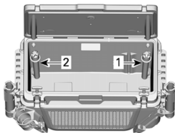
1. Vatteninlopp betes-/fisksump 2. Vattenutlopp betes-/fisksump
