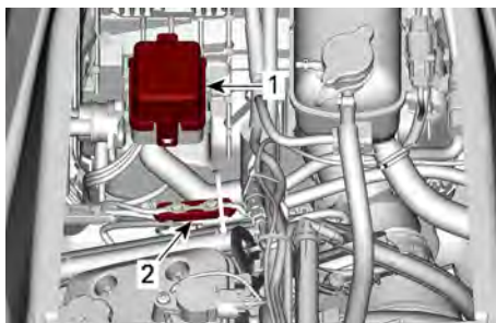
1. 保险丝盒 2. 主保险丝
