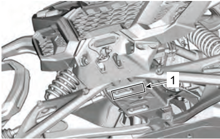
1. Hefgedeelte vooraan
