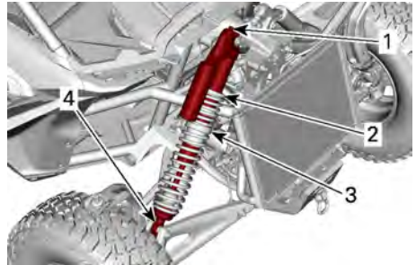
TYPISCH – VORDERRADAUFHÄNGUNG
