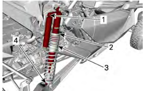
TYPISCH - HINTERRADAUFHÄNGUNG
