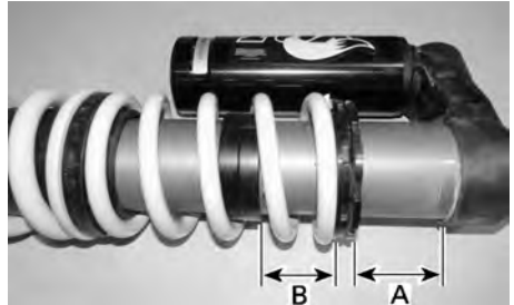
TYPISCH - CROSSOVER-EINSTELLUNG - HINTERER STOßDÄMPFER
