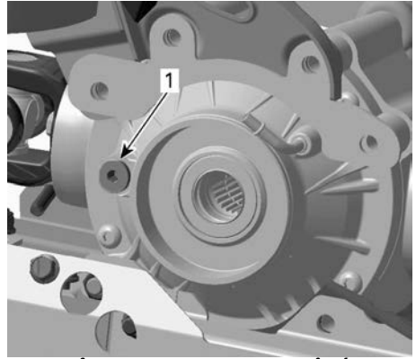
ENTRAÎNEMENT CENTRAL, CÔTÉ GAUCHE DU VÉHICULE
