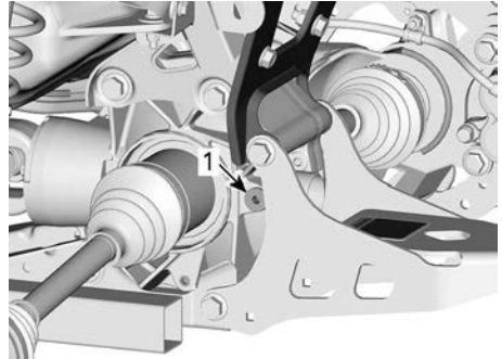
TRANSMISSION FINALE ARRIÈRE, CÔTÉ GAUCHE DU VÉHICULE
