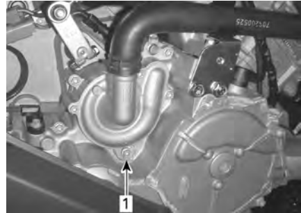
1. Tapón de drenaje de refrigerante
