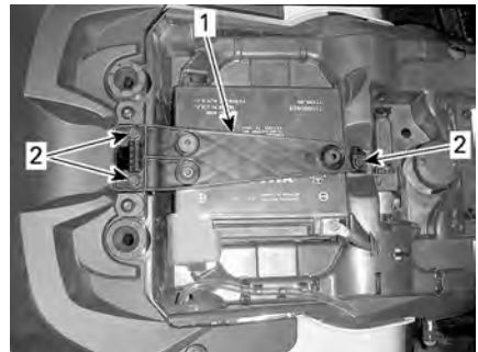
1. Correa de sujeción de la batería 2. Tornillos de sujeción
