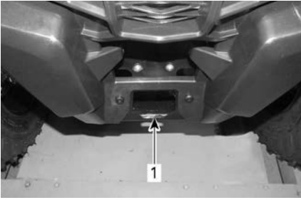
1. Gancho de recuperación delantero
