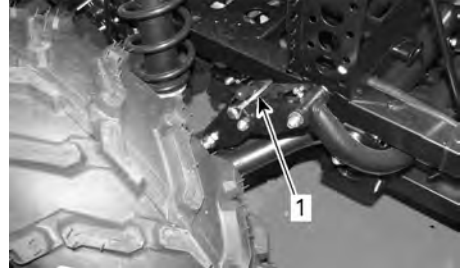
1. Pasador de la barra estabilizadora bloqueado
