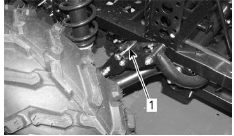
1. Pasador de la barra estabilizadora bloqueado
