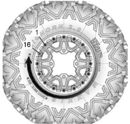
TYPIQUE - SÉQUENCE DE SERRAGE FINAL
