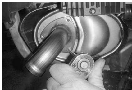
TYPIQUE - RETRAIT DU TUYAU ARRIÈRE
