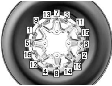
TYPIQUE - SÉQUENCE DE SERRAGE
