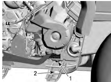
1. Tapón de drenaje magnético 2. Acceso a través del bastidor
