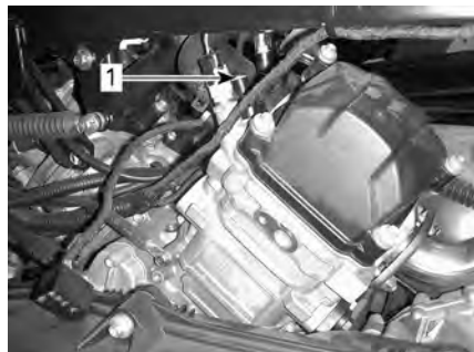
1. Tornillo de purga del cilindro trasero
