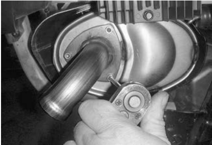
TYPISCH - ABGASROHR ENTFERNEN
