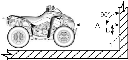
1. Lichtstrahlmitte
