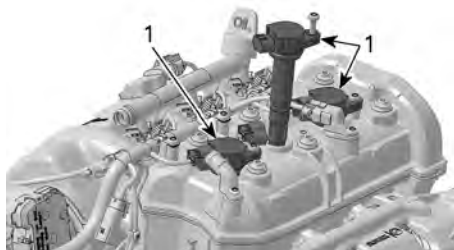
1. Tändspolar
