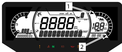
TÍPICO – CENTRAL DE INFORMAÇÕES – INDICADOR DE POSIÇÃO DO VTS
