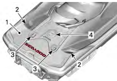
ウェイクボードラック用保持ブラケット
