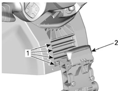
典型示例 - 转向柱调整锁栓固定
