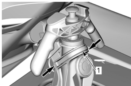
代表的な例 - パイロンを前方に押し、ロッキングクリップを解除し、取り外す
