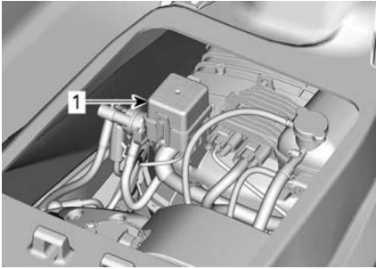
TYYPILLINEN 1. Sulakekotelo
