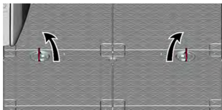
TIRER SUR LES POIGNÉES DE VERROUILLAGE
