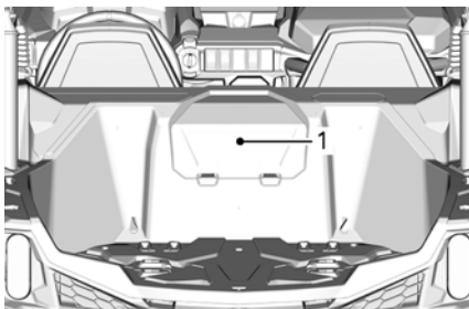
1. Kjølevæskebeholderens tilgangsdeksel
