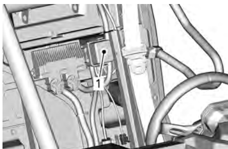
1. Zekeringsdoos achter
