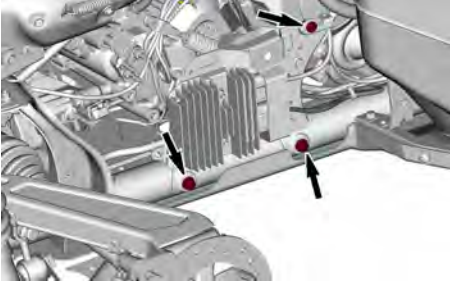
SCHROEVEN SPANNINGSREGELAAR
