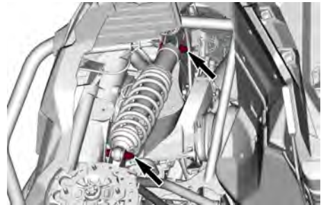
TYPISCH — BEVESTIGINGEN SCHOK-DEMPEMPEL VOOR
