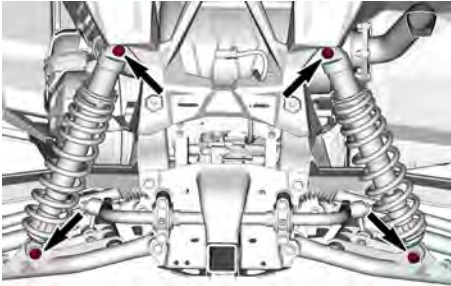
TYPISCH — BEVESTIGINGEN SCHOK-DEMPEMPER ACHTER
