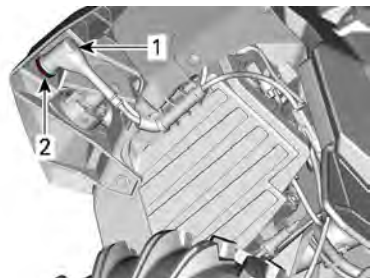
1. Conector eléctrico de la luz de posición 2. Tuerca de sujeción
