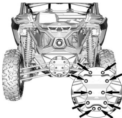
TÍPICO - BARRA ESTABILIZADORA DIANTEIRA
