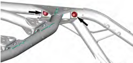
HINTERE, BEFESTIGUNGSELEMENTE
