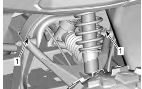
1. Fjädringsarmens smörjnipllar
