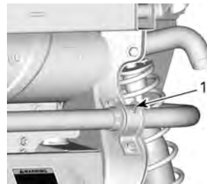
1. Smörjnippel på bussning för bakre krängningshämmare
