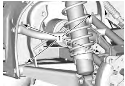
1. Smörjnipllar på bakre bärm
