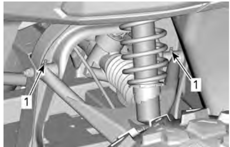
1. Jousitustukivarren rasvanipat
