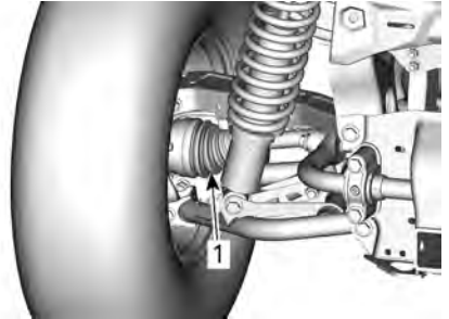
TYPISK - BAKRE HJULSIDE
