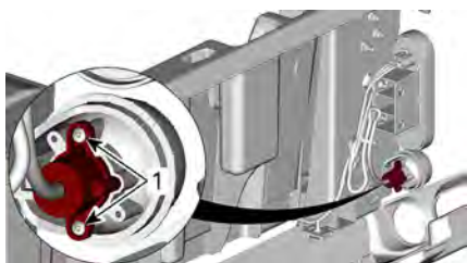
1. Viti di blocco
