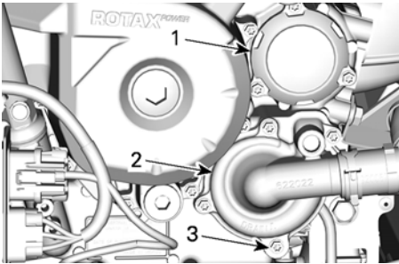
MOTORE V-TWIN
