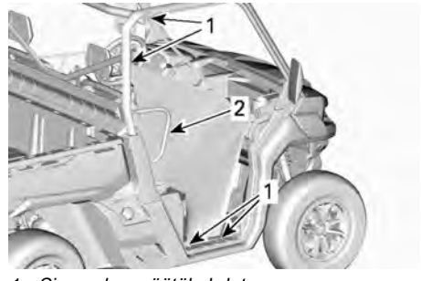
1. Sivuverkon säätökohdat 2. Olkasuoja
