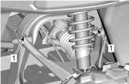
1. Jousitustukivarren rasvanipat
