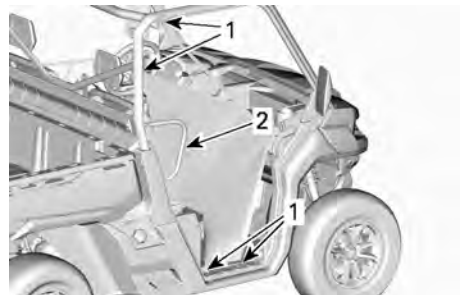
1. Seitennetz-Einstellungsorte
