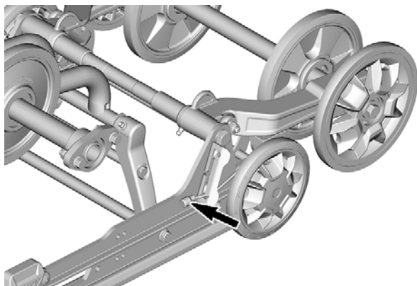
BAKRE FÖRHÖJNINGSLÅSINSTÄLLNING – LÅST POSITION
