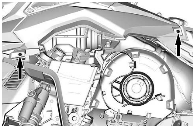
VASEN PUOLI
