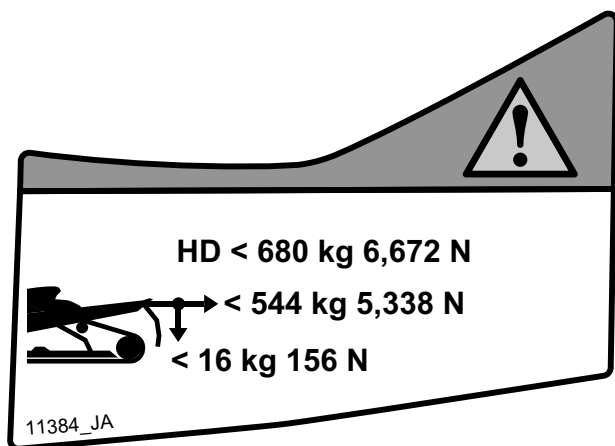
最大けん引能力 - 警告ラベル
