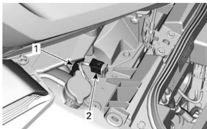
1. 診断コネクター (BUDS2用)
