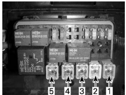
FUSIBILI A CAPSULA - SCATOLA FUSIBILI SINISTRA
