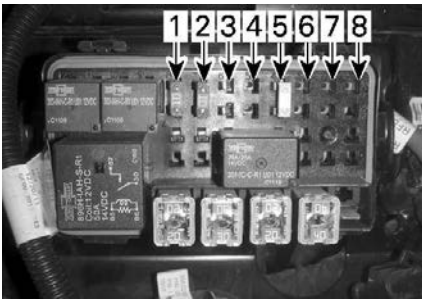
保险丝 - 右侧保险丝盒
