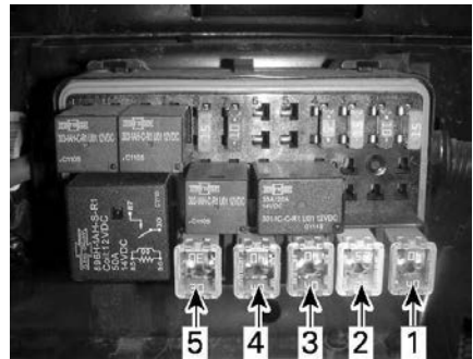
JCASE 保险丝 - 左侧保险丝盒
