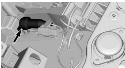
DC56 - 后客户配件电路 - 乘客座椅下
