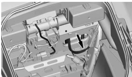
DC12 - 前客户配件电路 - 储物舱后方 2. 横向检修盖后方。
