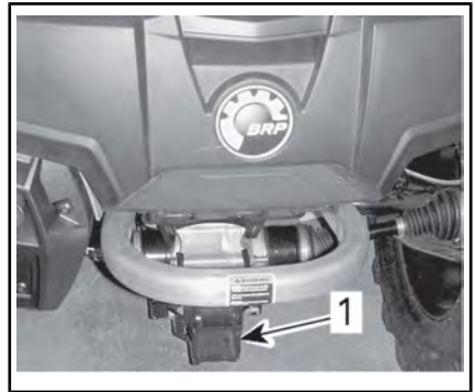
1. Trailer hitch Anhängerkupplung
