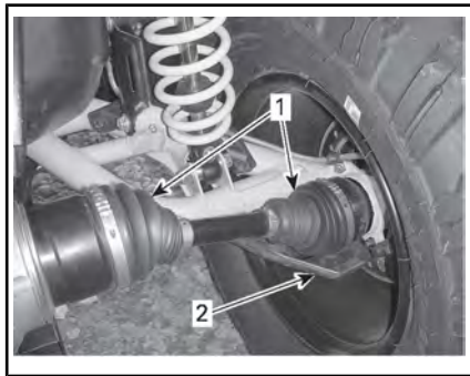
TYPISCH — FAHRZEUGRÜCKSEITE
