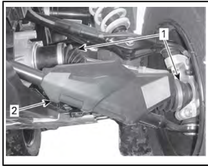
TYPISCH — FAHRZEUGVORDERSEITE
