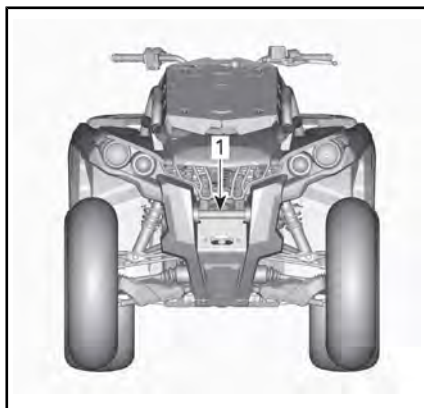
1. Vorderer Verzurrpunkt
