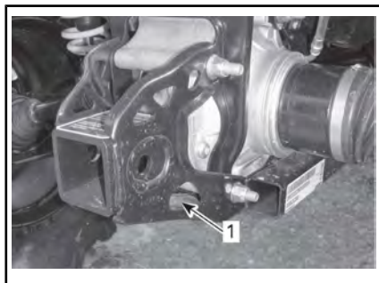
1. Hinterer Verzurrpunkt
