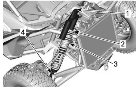
TYPISK – FJÆRING FORAN
