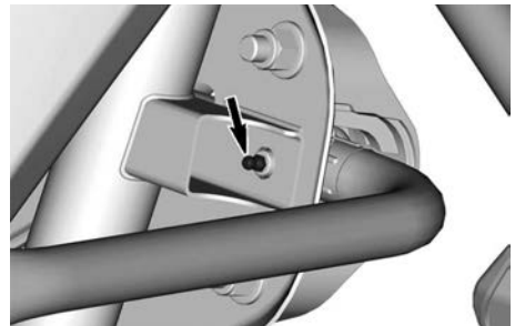
BAKRE STABILISATORSTAG - VENSTRE SIDE - TYPEBILDE
