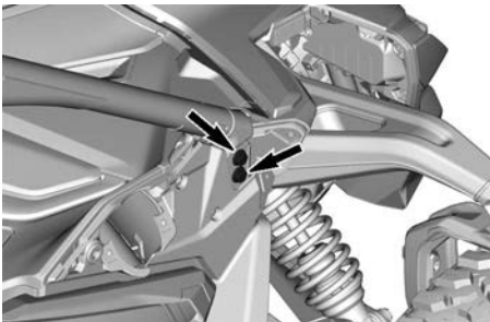
FREMRE FESTE PUNKTER – TYPEBILDE
