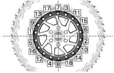
SITUAZIONE TIPICA - SEQUENZA DI SERRAGGIO
