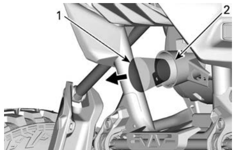
VITI DELLO SCARICO - LATO DESTRO (CONFIGURAZIONE TIPICA)
