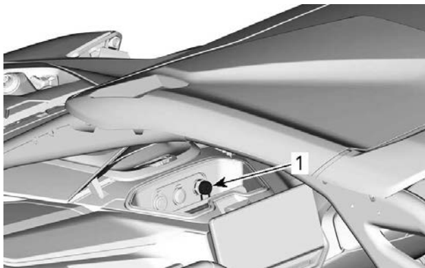
1. Port USB écran tactile
