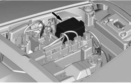
VOORSTE ZEKERINGDOOS
