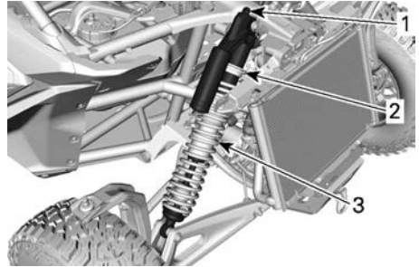
TYPISCH - VOOROPHANGING
