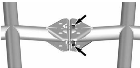
BEVESTIGINGEN MIDDEN
