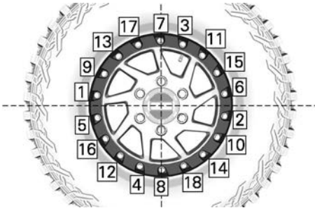
TYPISCH - AANDRAAIVOLGORDE
