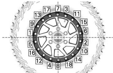
TYPISCH - AANDRAAIVOLGORDE
