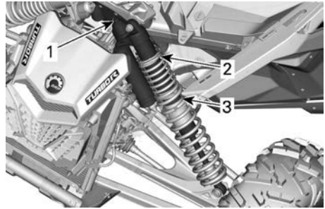
GEWOONLIJK - ZONDER TERUGVEERDEMPING - WIELOPHANGING VOÓR
