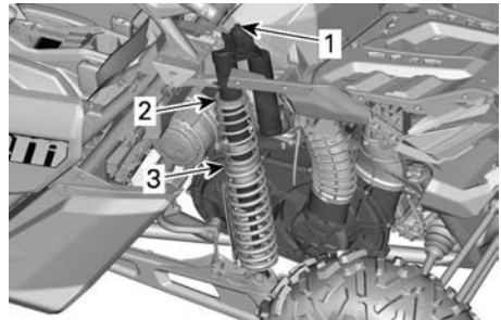
GEWOONLIJK - ZONDER TERUGVEERDEMPING - WIELOPHANGING ACHTER
