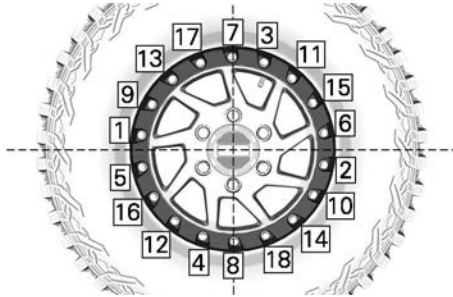
TYPISCH - AANDRAAIVOLGORDE
