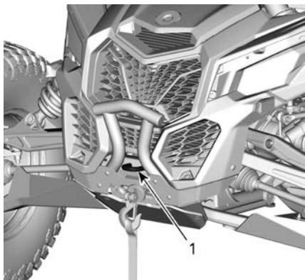
1. 前部挂挂钩
