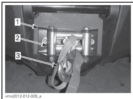
1. Cabestrante 2. Guiacabos de rodillos 3. Gancho del cabestrante
