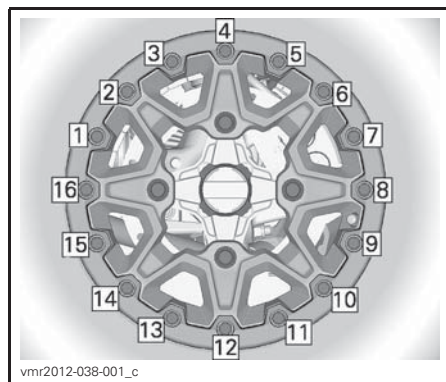
SECUENCIA DE APRIETE FINAL
