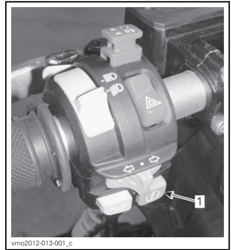
TÍPICO 1. Botón de arranque del motor
