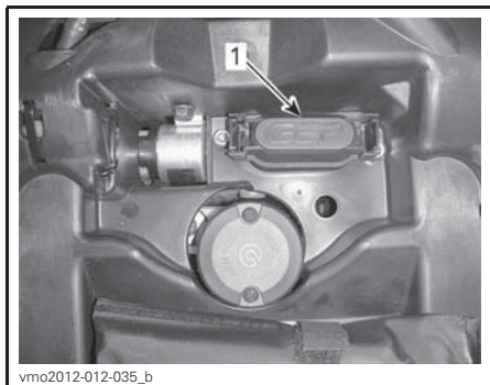
1. Tapa del portafusibles trasero
