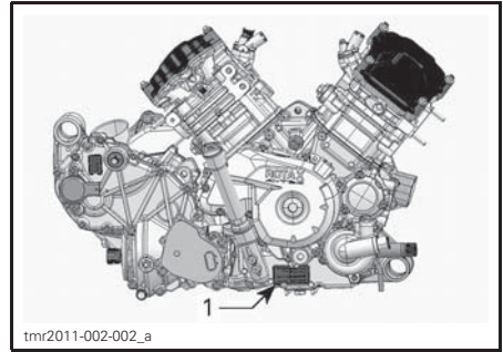
TÍPICO - LATERAL DERECHO DEL MOTOR 1. Número de identificación del motor (E.I.N.)
