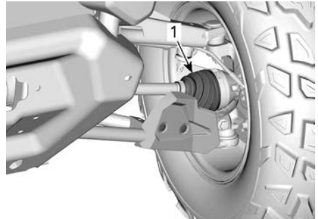
1. Soufflets d'arbre de transmission extérieur
